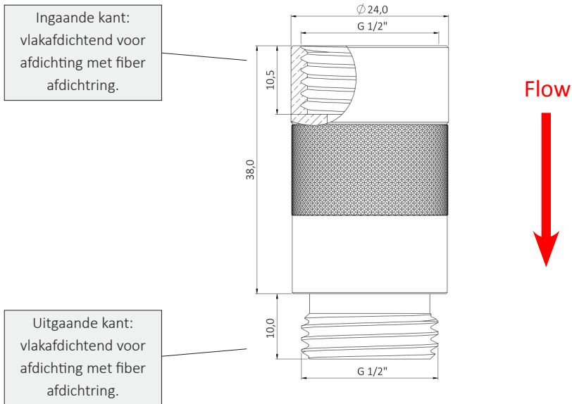
Afbeelding: HL2024 Shower (afmetingen in mm)
